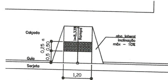
○ Detalhe das rampas de acessibilidade
