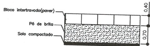
○ Detalhe camadas calçadas
